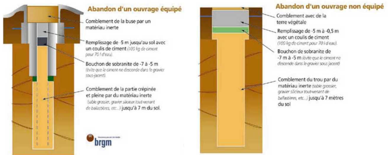
Figure 40 : Prescriptions pour l'abandon d'un forage
