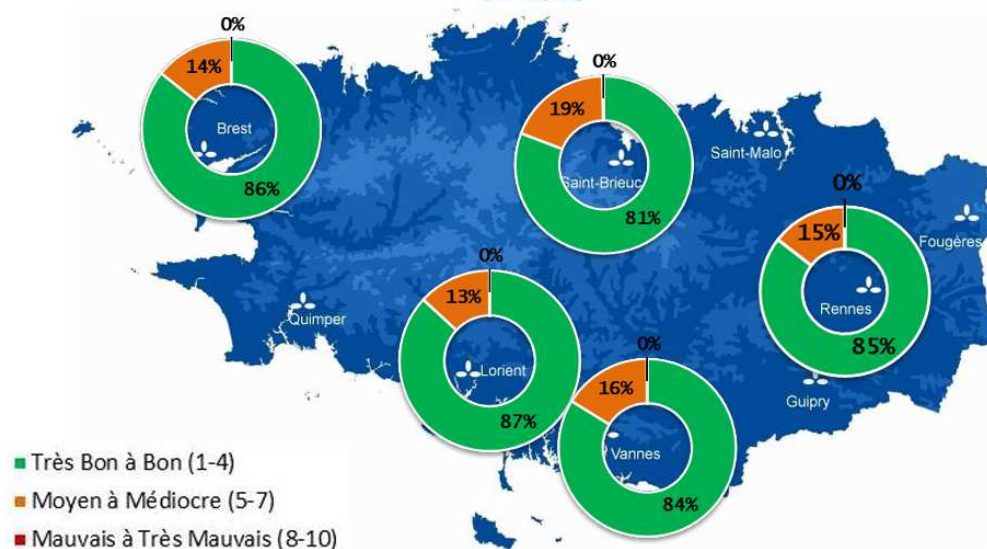
Figure 28 : Qualité de l'air en Bretagne
