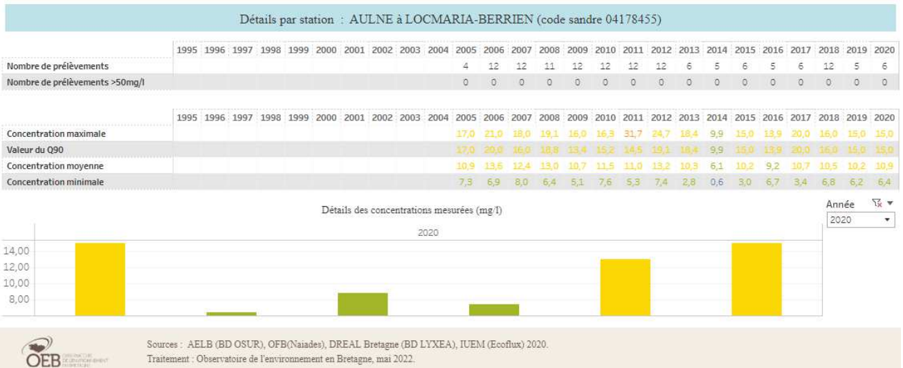
Figure 36 : Concentration en nitrates (mg/L) au niveau de l'Aulne à LOCMARIA BERRIEN.
