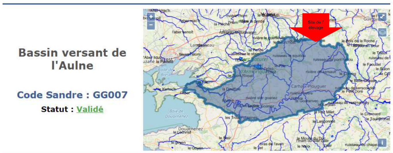
Figure 34 : Bassin versant de l'aulne
