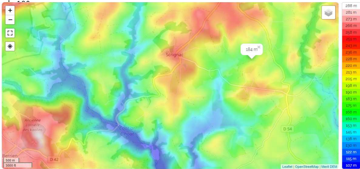
Figure 43 : Carte du Relief de la zone d'études
