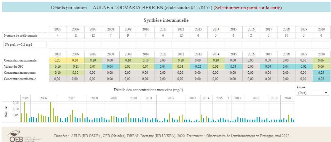
Figure 38 : Concentration en phosphore total (mg/L) au niveau de l'Aulne à LOCMARIA BERRIEN.
