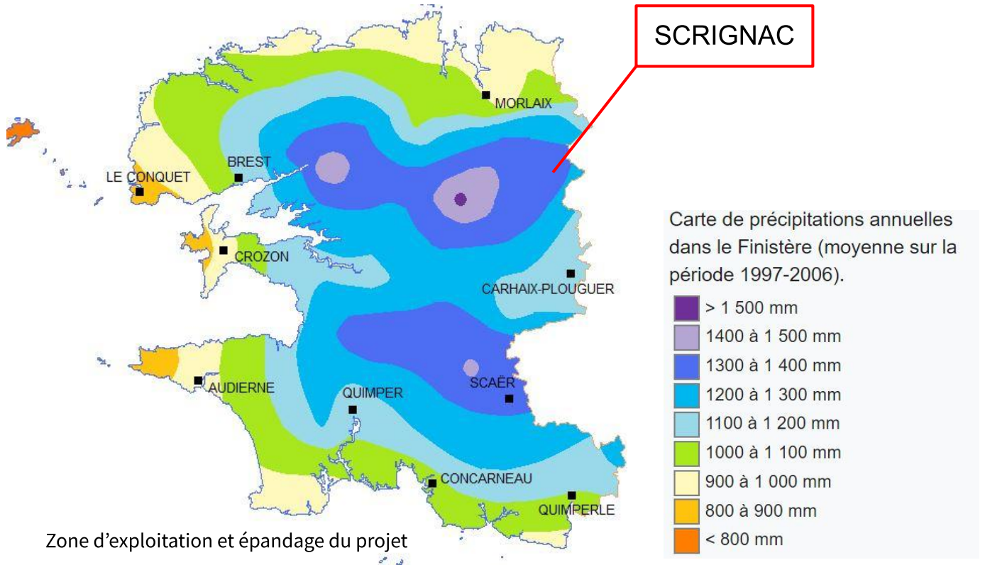
Figure 25 : Précipitations moyennes annuelles en Finistère entre 1997 et 2006
