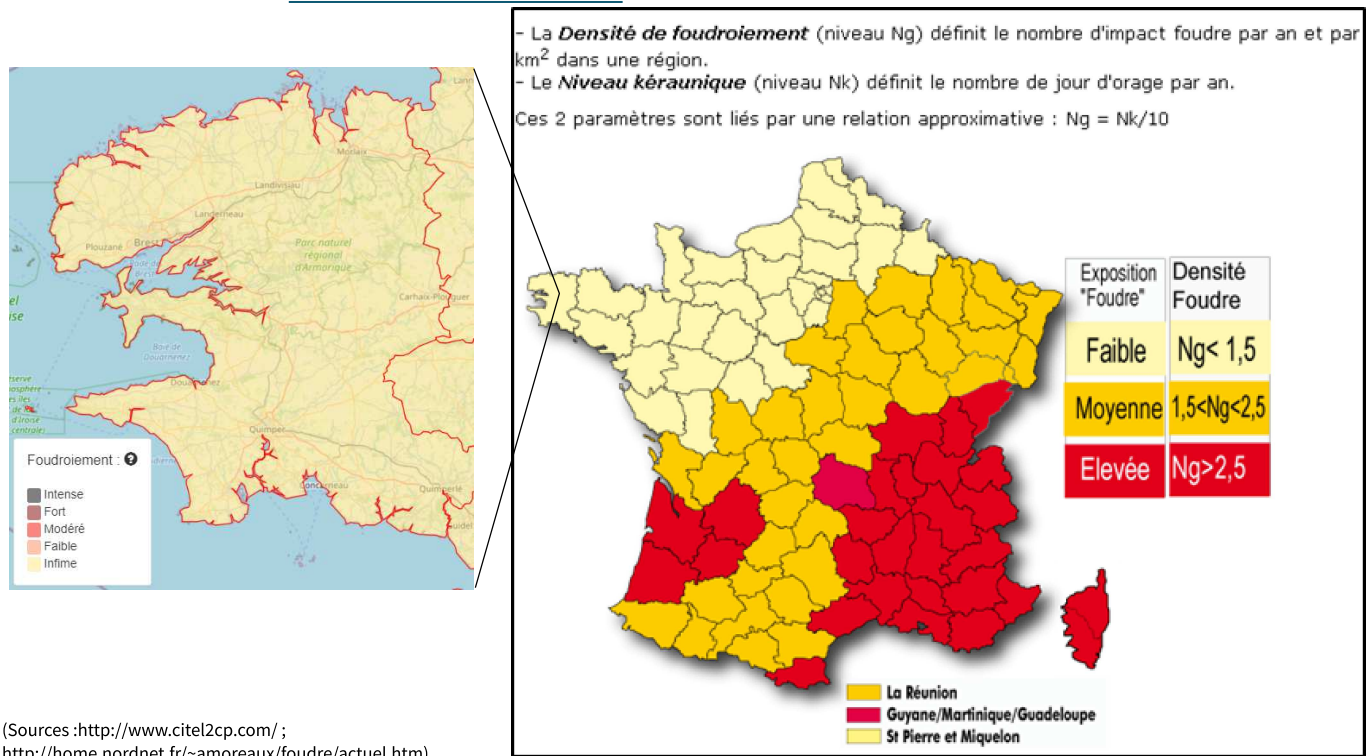
Figure 27 : Zone de foudroiement et niveau kéraunique en France
