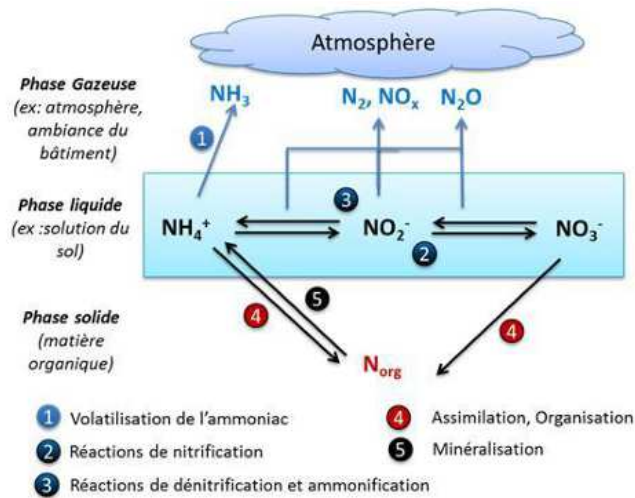
Figure 76 : Schéma simplifié des mécanismes conduisant à la formation des gaz azotés d'après l'ADEME (2012)
