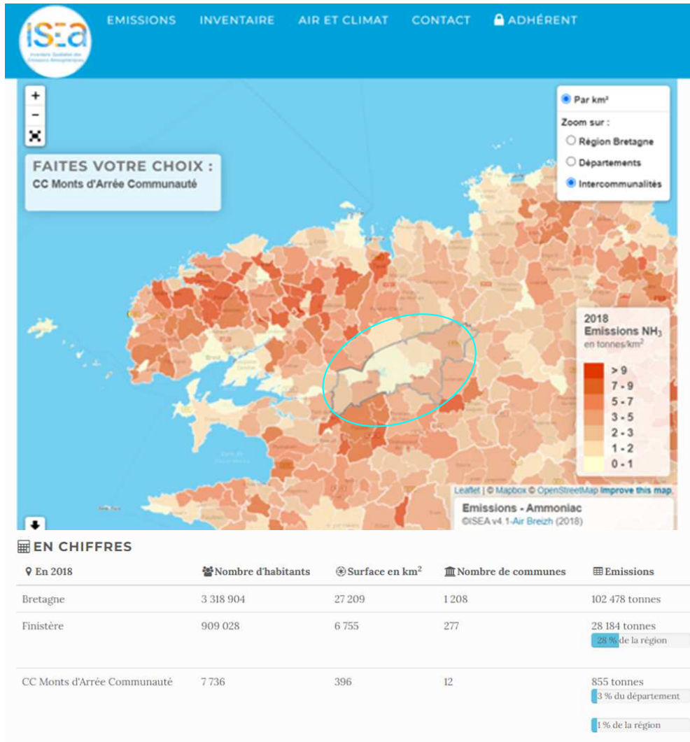
Figure 29 : Qualité de l'air en Bretagne
