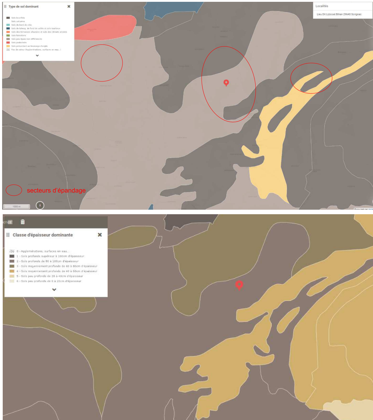
Figure 32 : Types et épaisseurs des sols sur la zone d'exploitation
