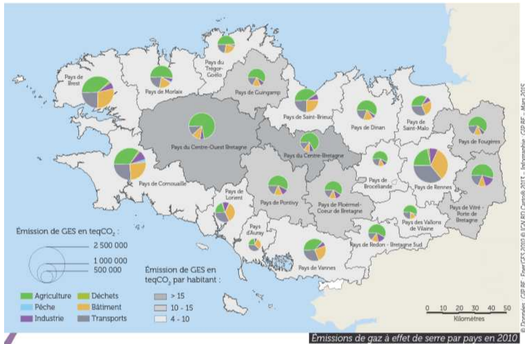
Figure 70 : Émissions de GES en BRETAGNE
