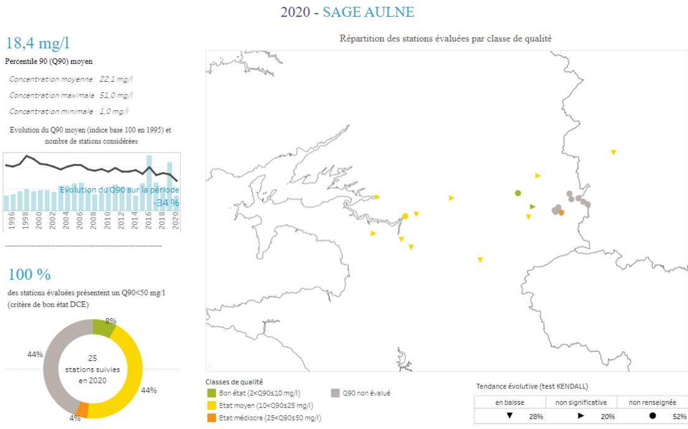
Figure 35 : Concentration en nitrates (mg/L) au niveau de l’Aulne
