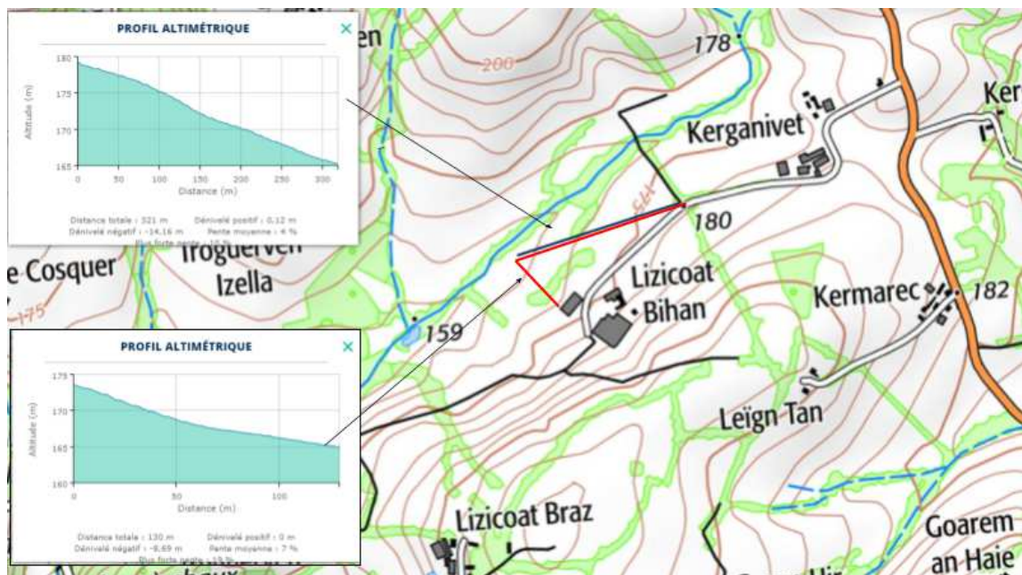
Figure 44 : Carte Topographique et profil du Relief de la zone d'étude
