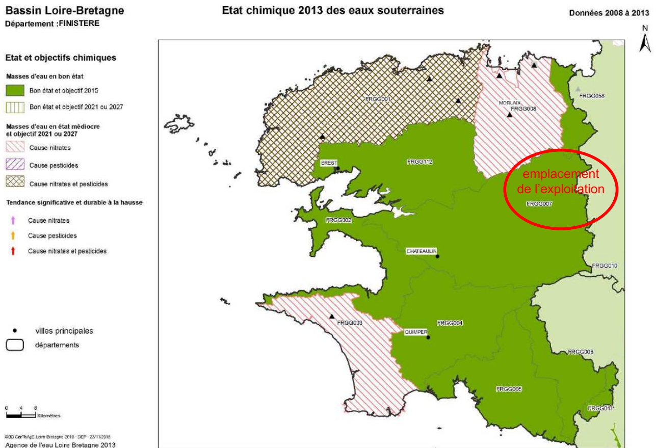
Figure 39 : Etat chimique 2013 des eaux souterraines en Finistère
