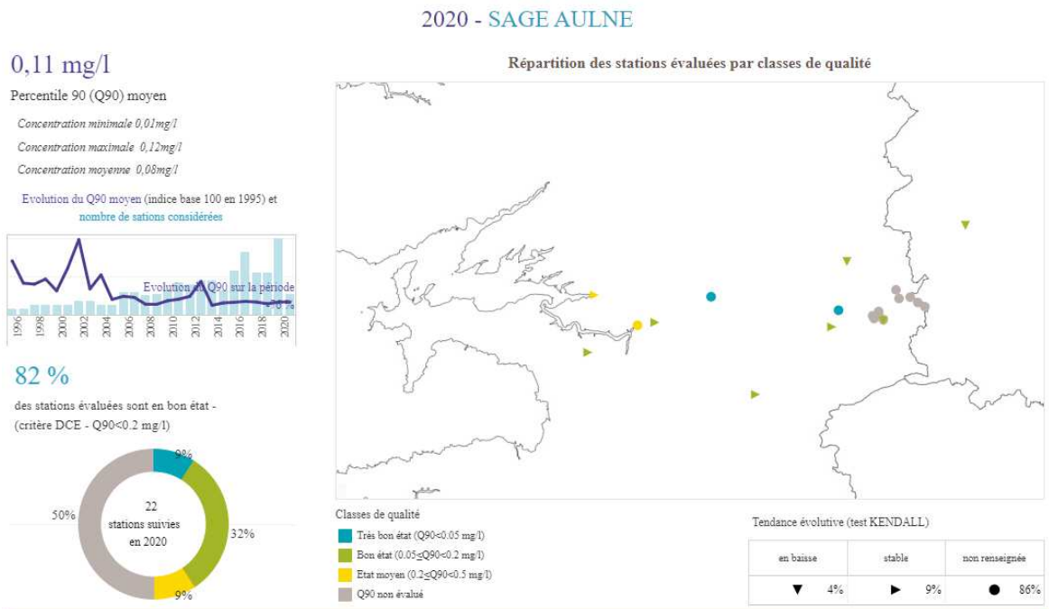
Figure 37 : Concentration en phosphore total (mg/L) au niveau de l'Aulne
