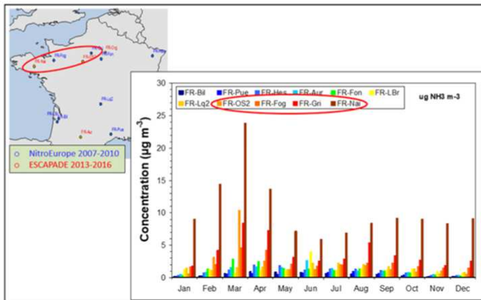
Figure 78 : Variabilité mensuelle des concentrations en NH3 en différents points de mesures (Fauvel et al., 2019).
